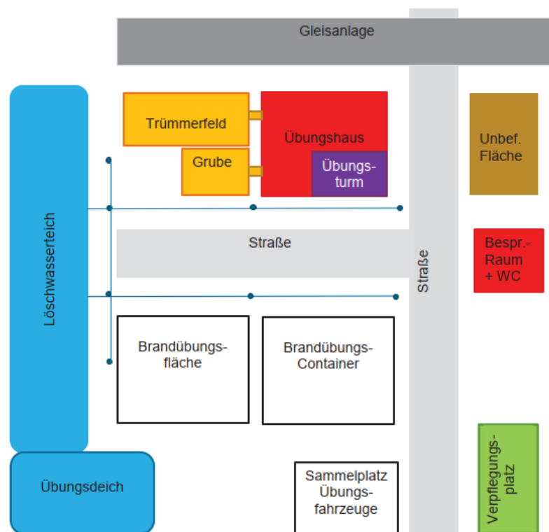
Abbildung 28: Beispielhafter Aufbau einer Übungsanlage 60
