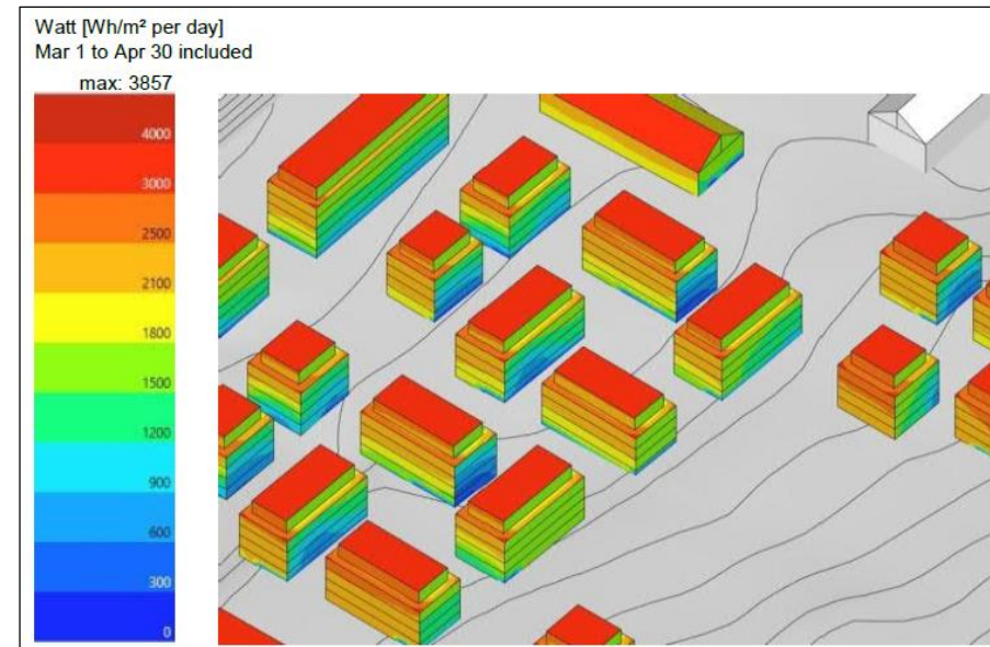
Abb.: Simulation solare Einträge im Mittel über den Betrachtungszeitraum Quelle: Klimagerechte Bauleitplanung für die Region Mittlerer Oberrhein, S. 47.
