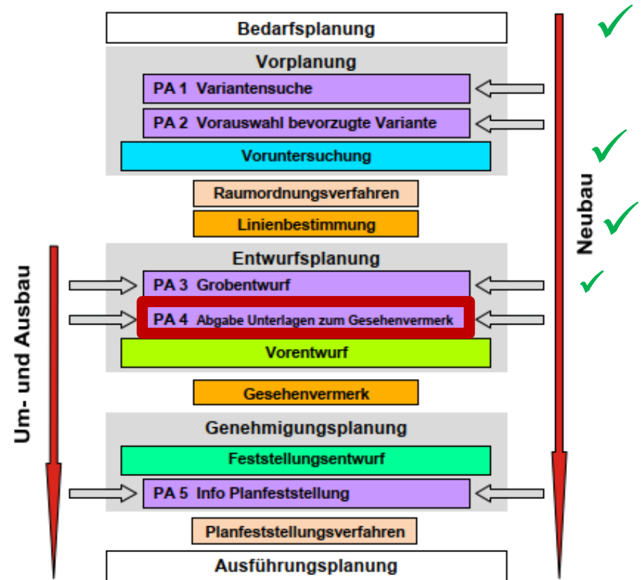
Abb.: Planungsprozess, Quelle: RE 2012
