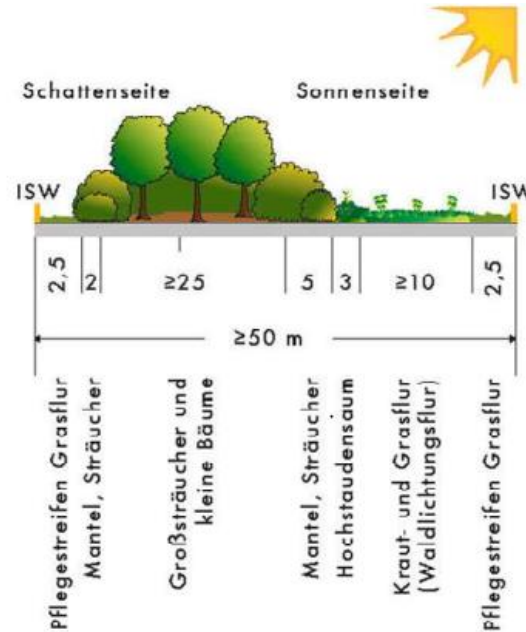
a) Grünbrücke – Standardlösung Seitenansicht
