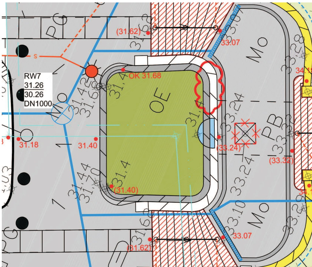
Lageplanausschnitt Brunnenbecken
