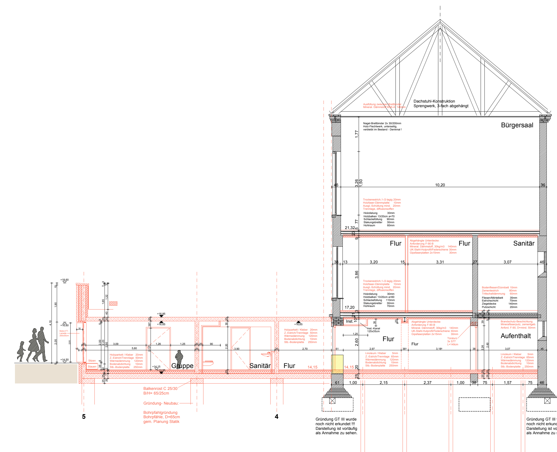
Schnitt S-08 Achse B - C Kita / Hort / Bürgersaal
