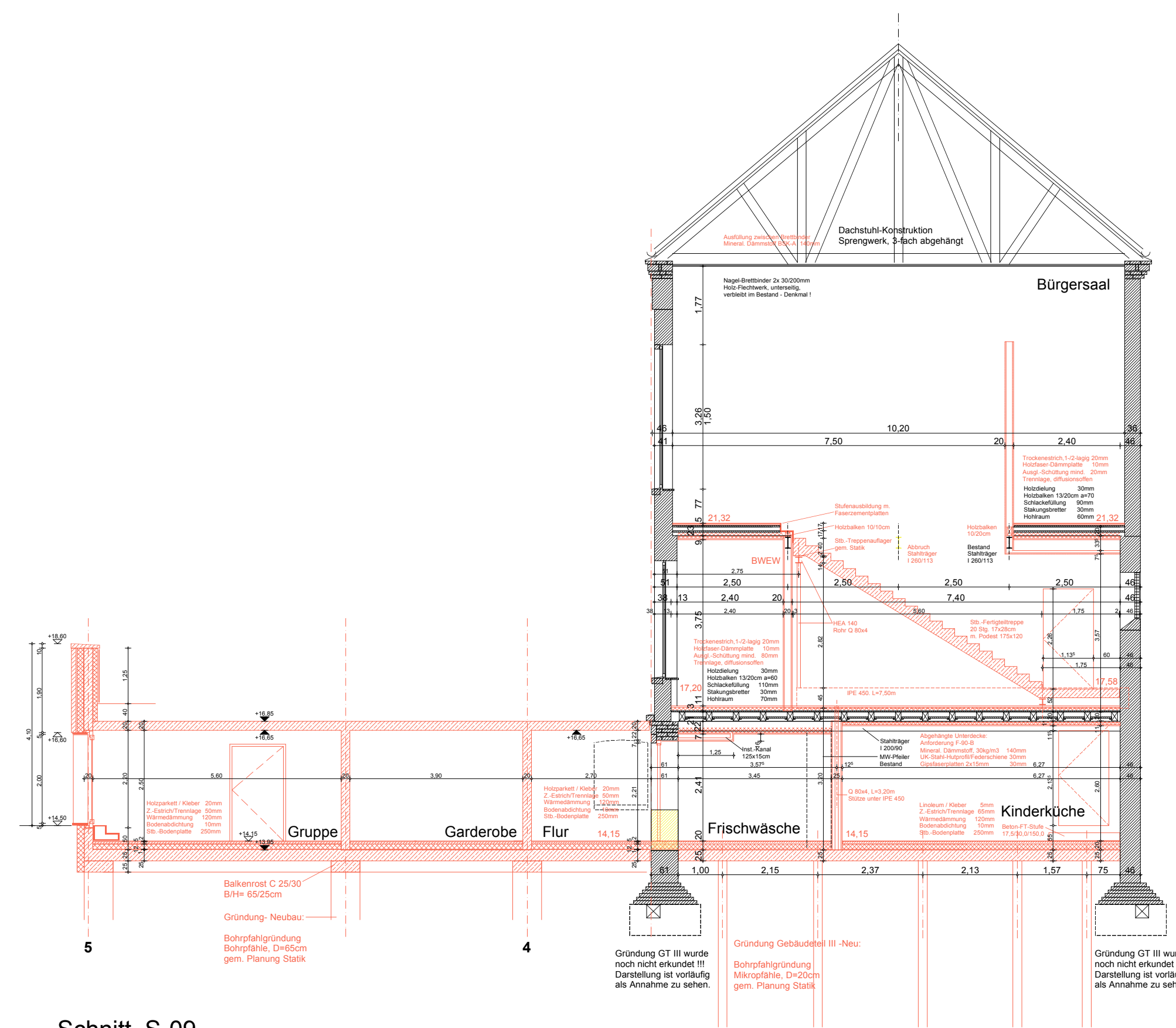
Schnitt S-09 Achse B - C Kita - Kinderküche - Treppe - Bürgersaal
